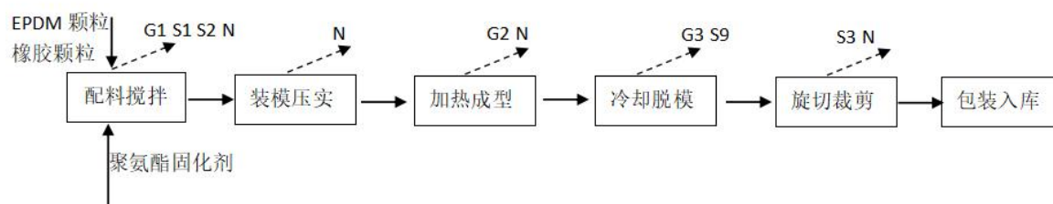
图 2-3 营运期橡胶地垫卷材生产工艺流程及产污环节图
