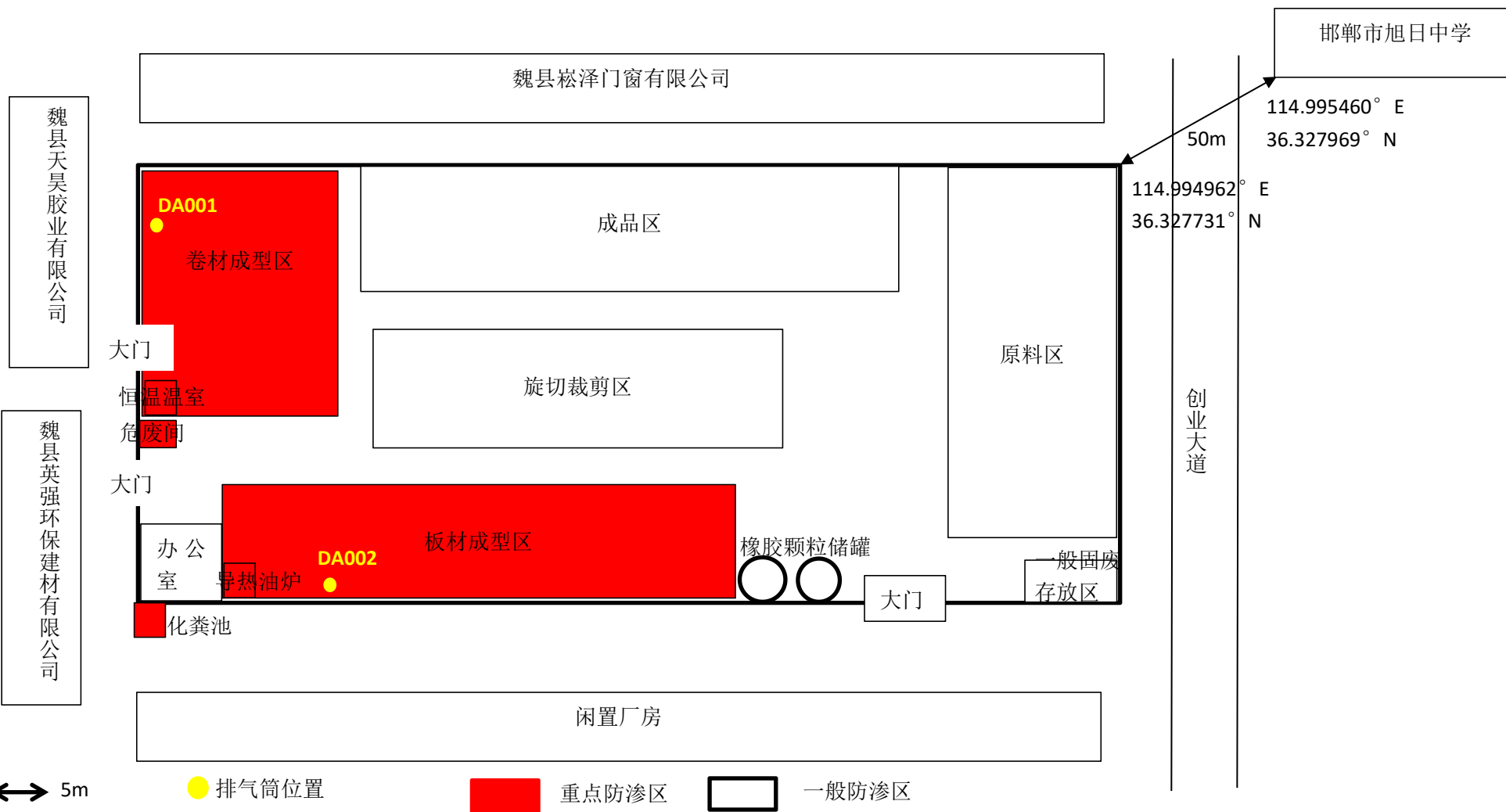
附图 3 厂区平面布置及分区防渗示意图
